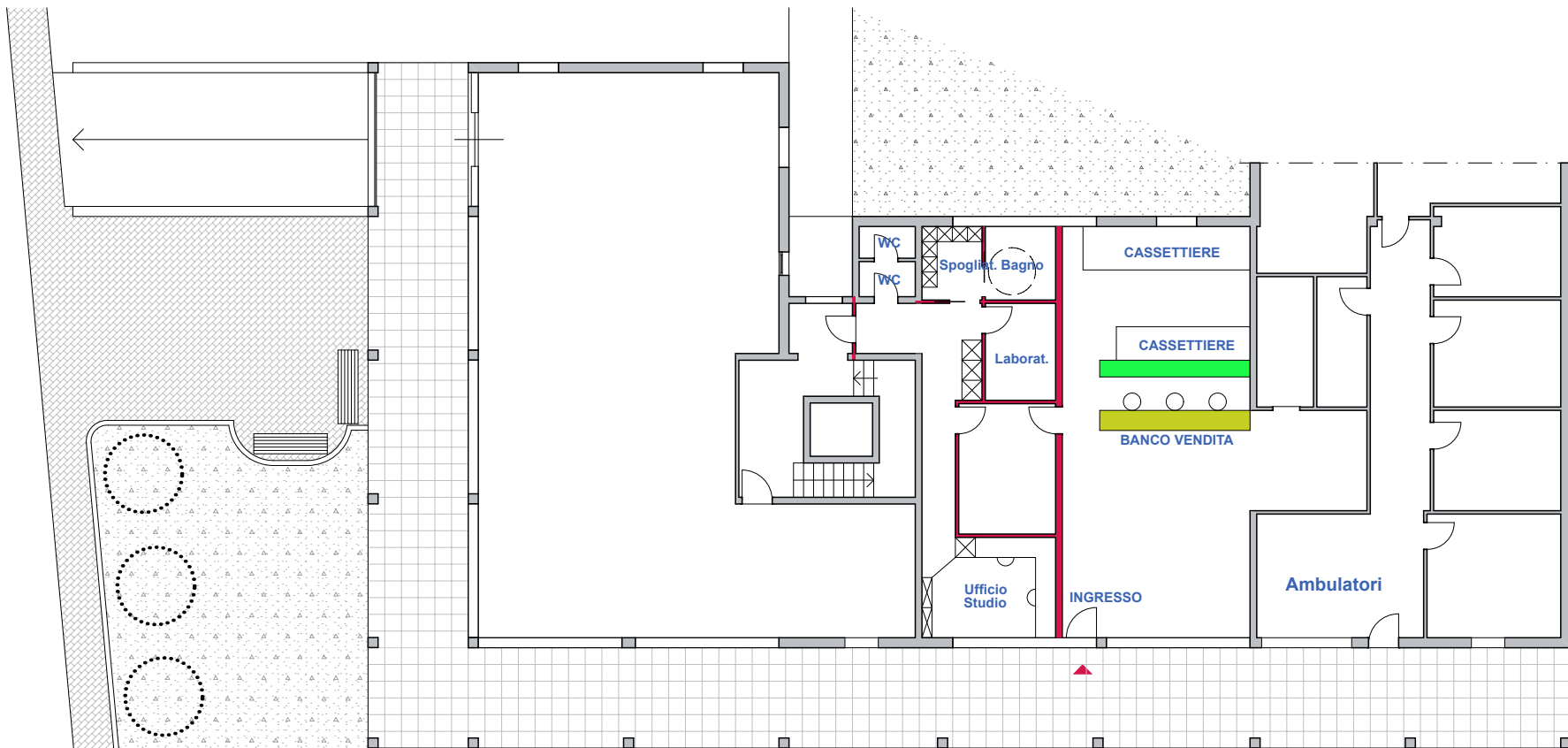
PIANTA PIANO TERRA Progetto fase transitoria - 1:200
