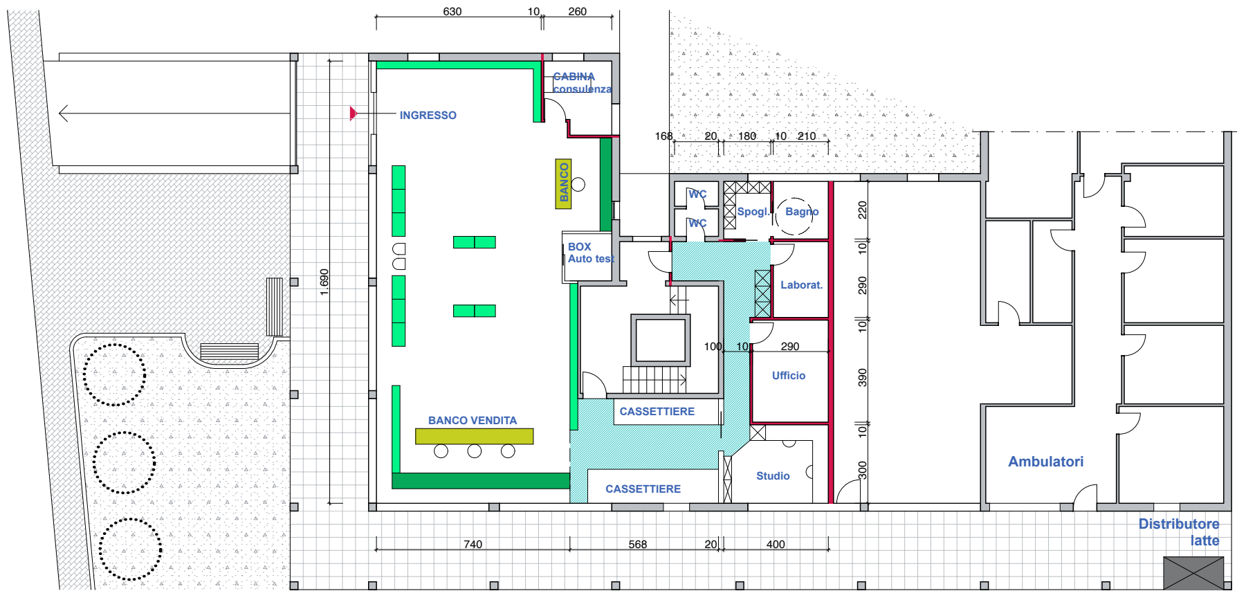
PIANTA PIANO TERRA Progetto - 1:200
