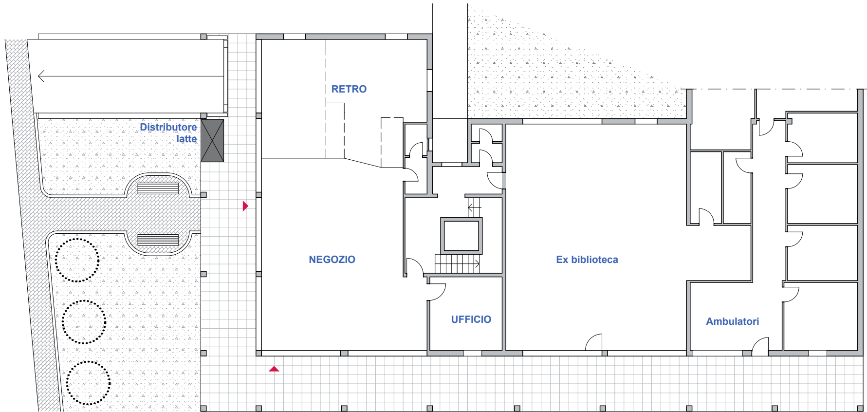
PIANTA PIANO TERRA Stato di fatto - 1:200
