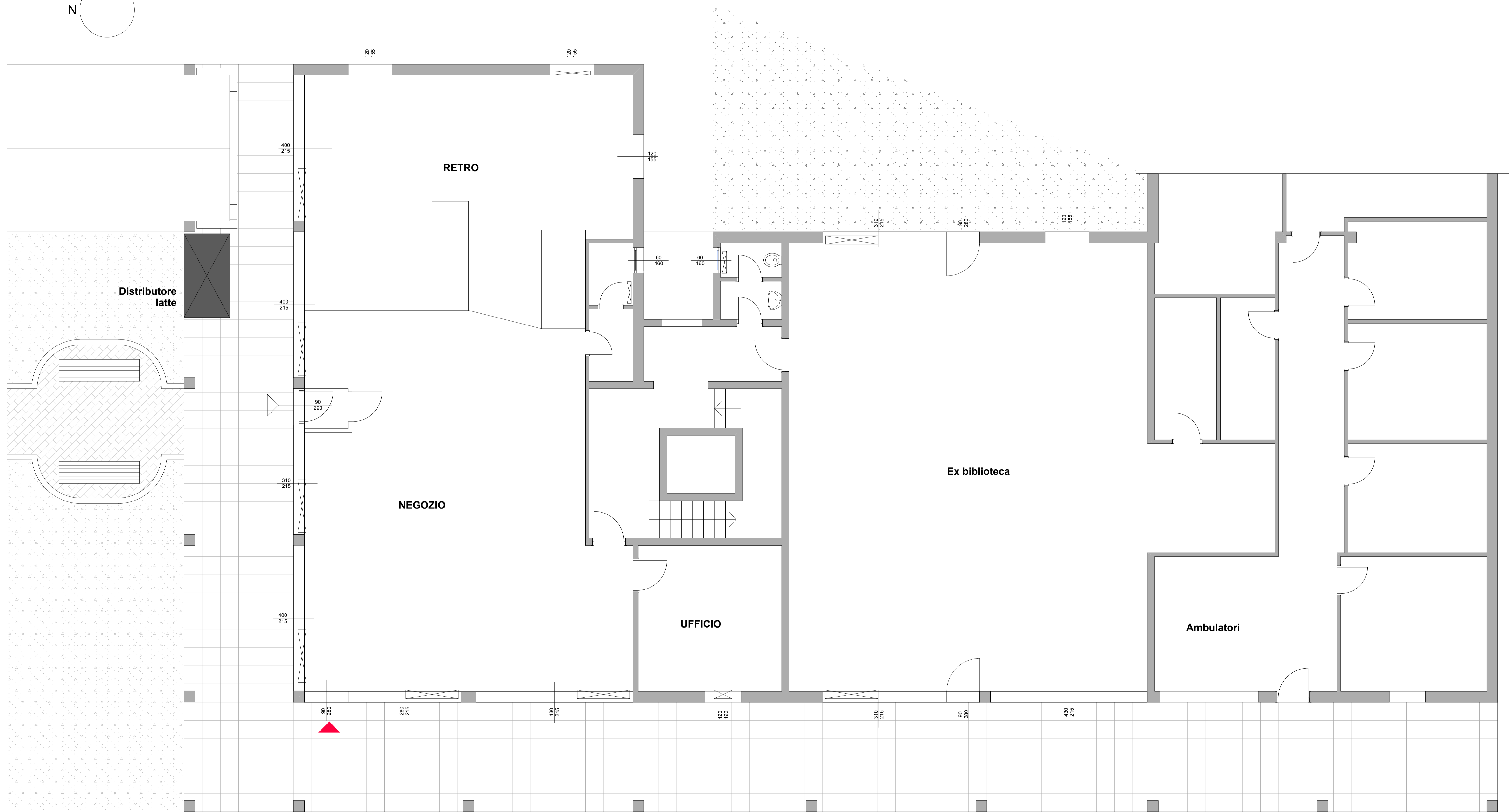
PIANTA PIANO TERRA - Stato di fatto - 1:50
