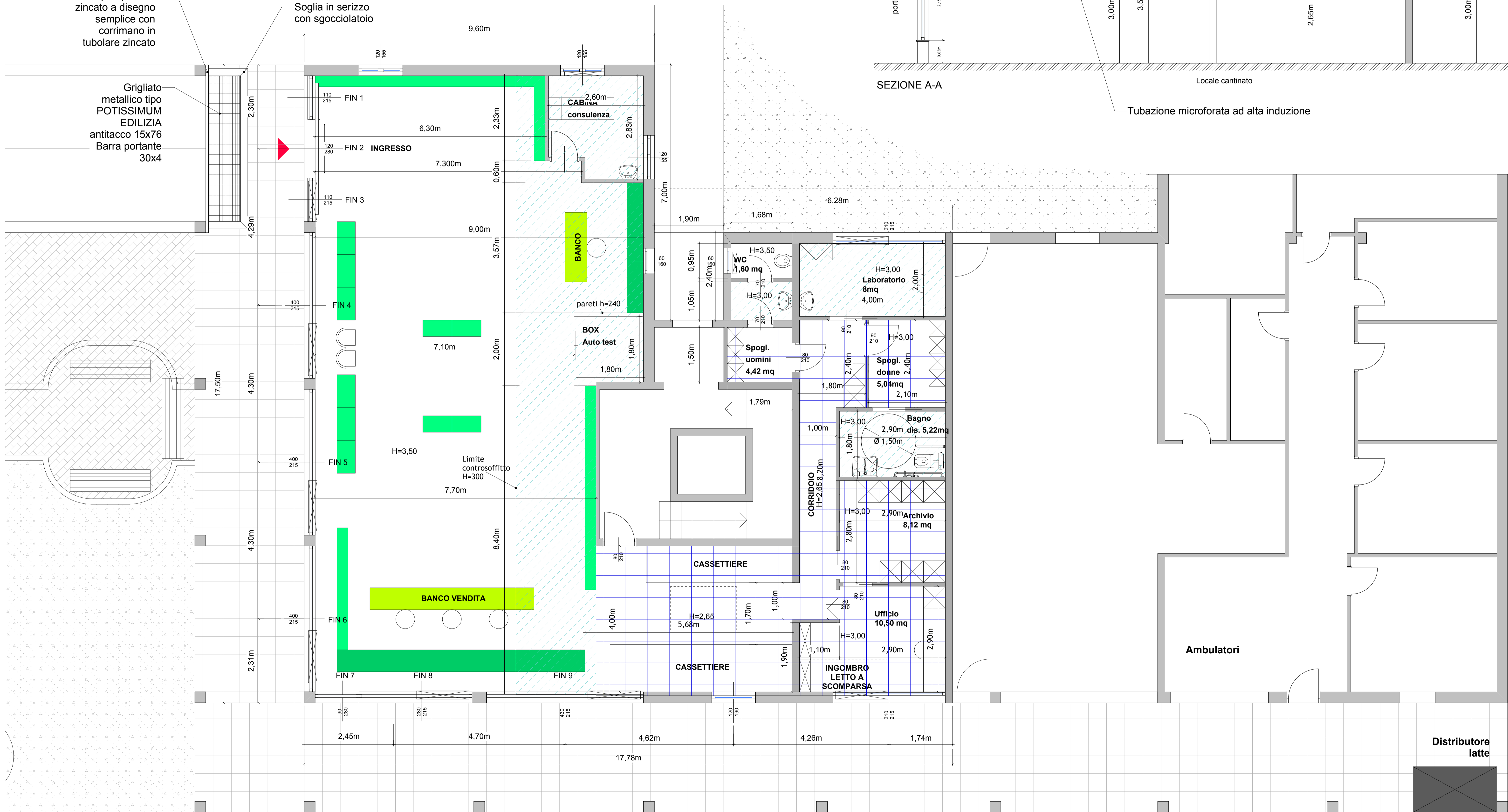
PIANTA PIANO TERRA - Progetto - 1:50
